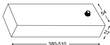
ΔΙΑΣΤΑΣΕΙΣ ΚΟΥΤΙ ΤΡΟΦΟΔΟΤΙΚΟΥ BOX FOR DRIVER DIMENSIONS
