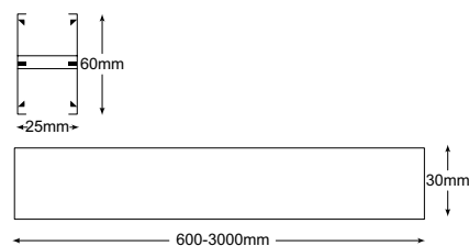
ΔΙΑΣΤΑΣΕΙΣ ΦΩΤΙΣΤΙΚΟΥ LUMINAIRE DIMENSIONS
