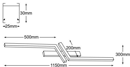
ΔΙΑΣΤΑΣΕΙΣ ΦΩΤΙΣΤΙΚΟΥ LUMINAIRE DIMENSIONS
